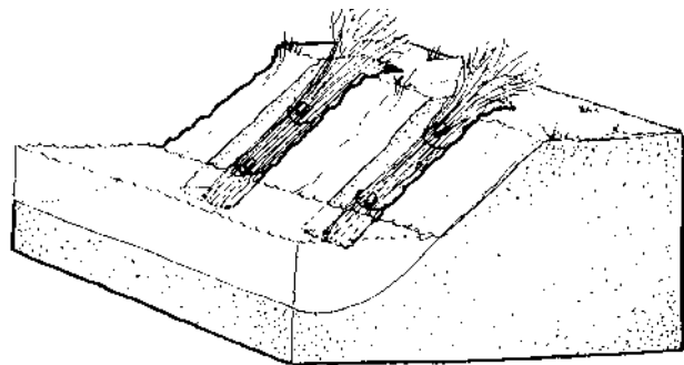
Brush Layer
