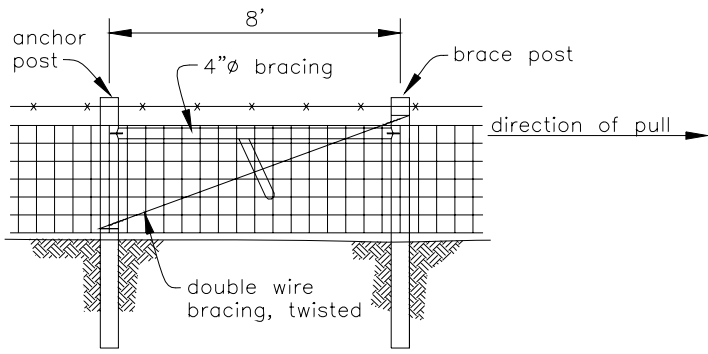
1-SPAN END
